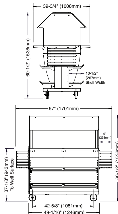
HFT2SYS-300 (Deluxe)
