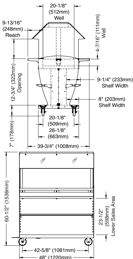
HFT2SYS-300 (Standard)
