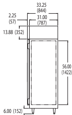
VF-1, VF-2, VF-3 SIDE VIEW
