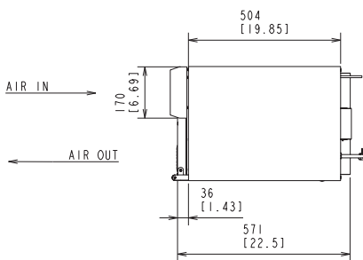
TOP DIMENSIONS
