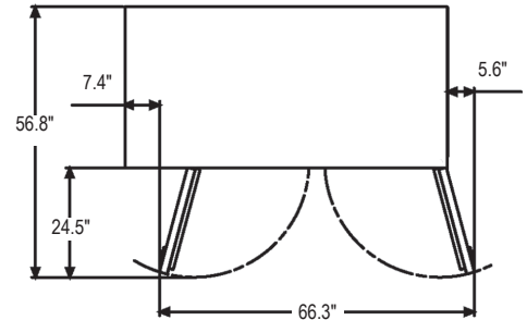
DOOR SWING
